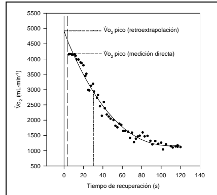
Figura 1. Curva de recuperación del consumo de oxígeno medida directamente (respiración a respiración) durante el período de recuperación inmediato tras una prueba máxima de 400 m. Se indican la curva de regresión y el valor pico \text{VO}_2 medido directamente y calculado por retroextrapolación.
